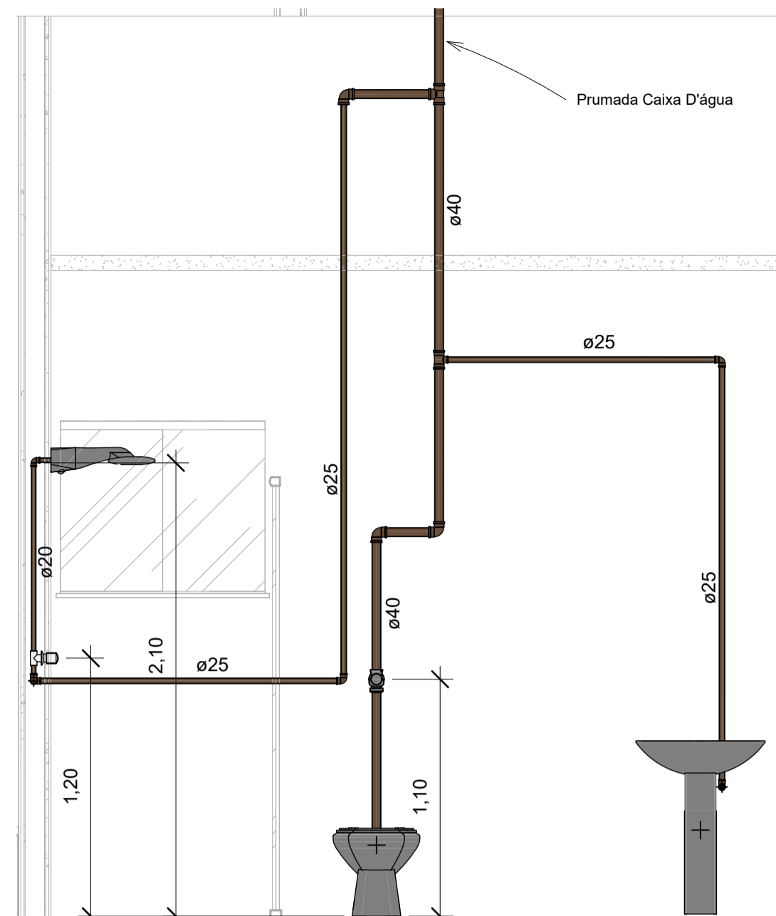
7 AF Banheiro Área Gourmet 1 : 25
