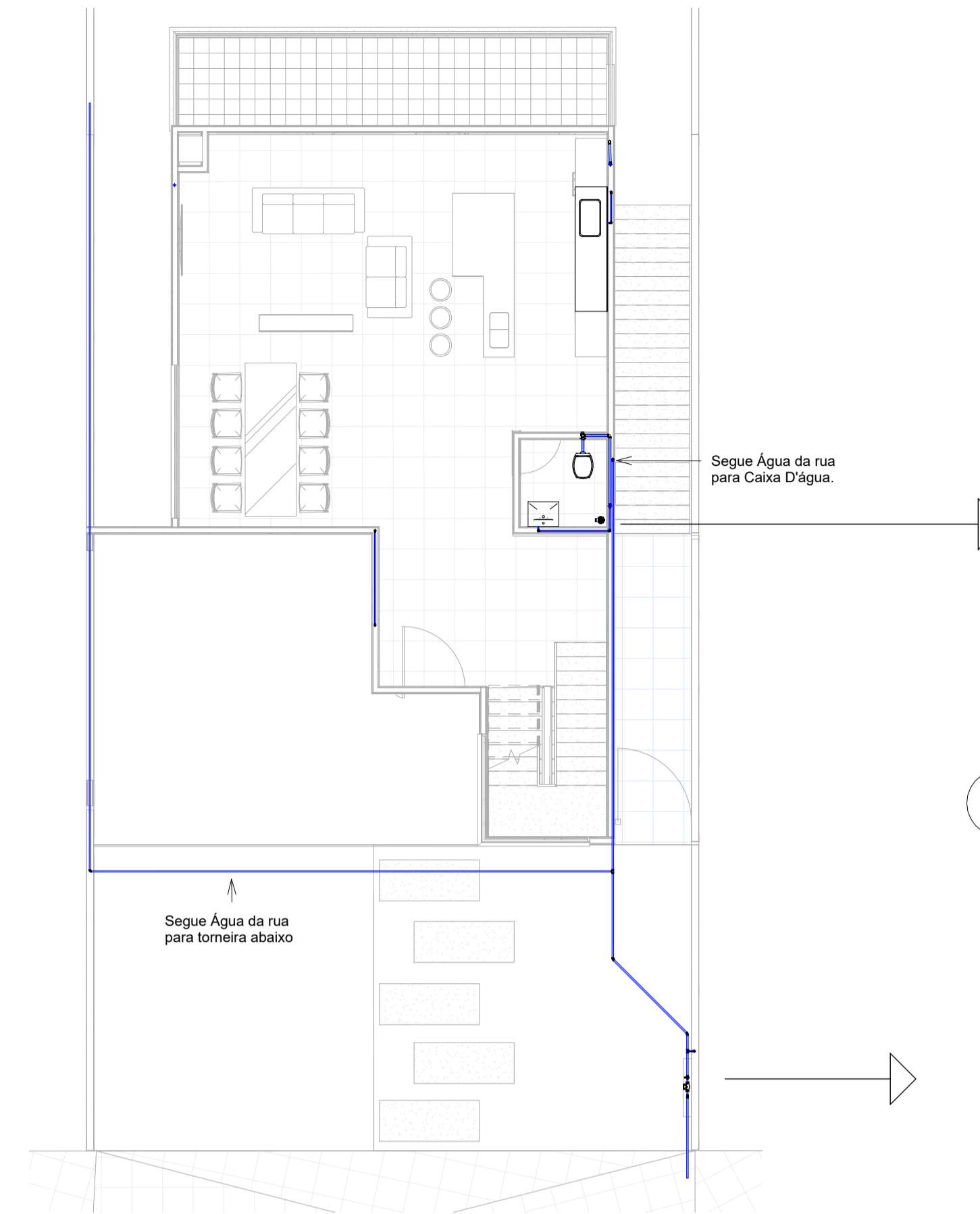
2 PAV. TERREO 1 : 100
