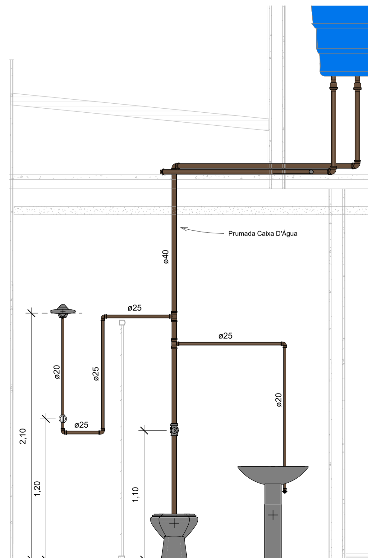
4 AF Banheiros Superior 1 : 20
