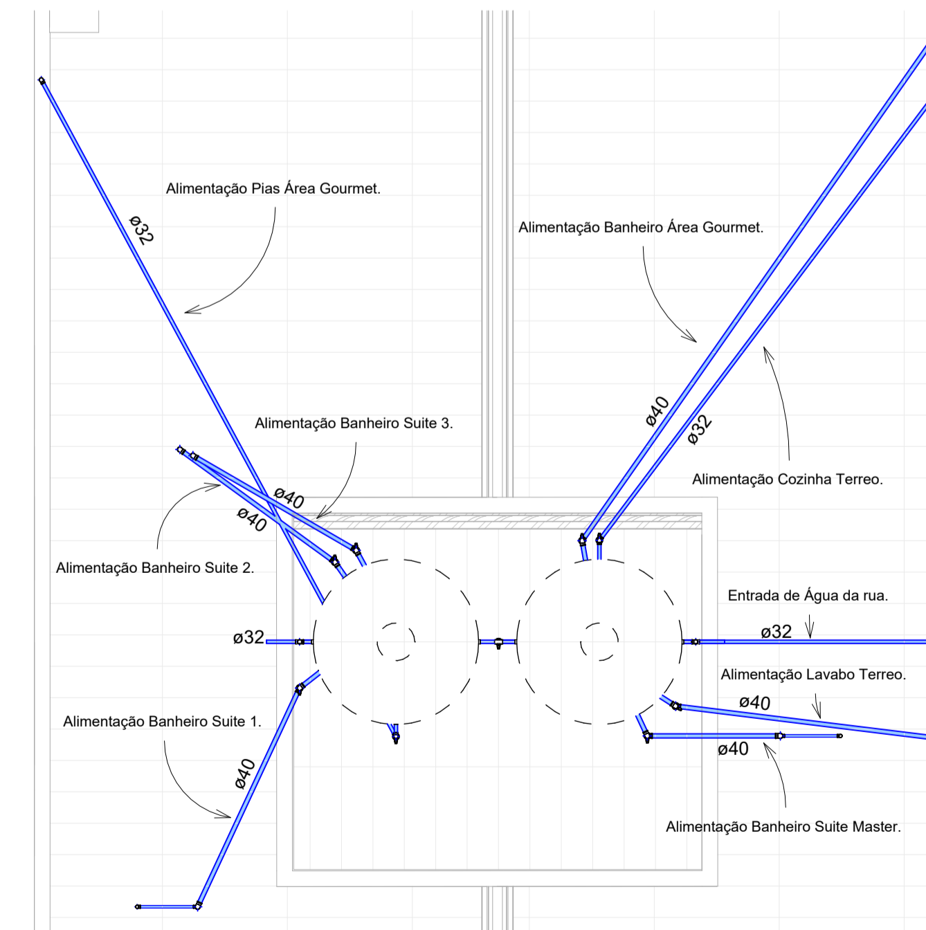
9 BARRILETE 1 : 50
