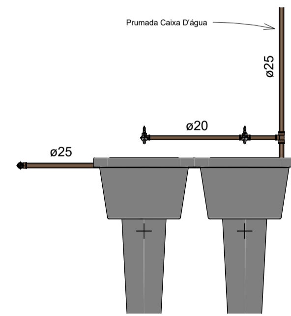
8 AF Lavanderia 1 : 20
