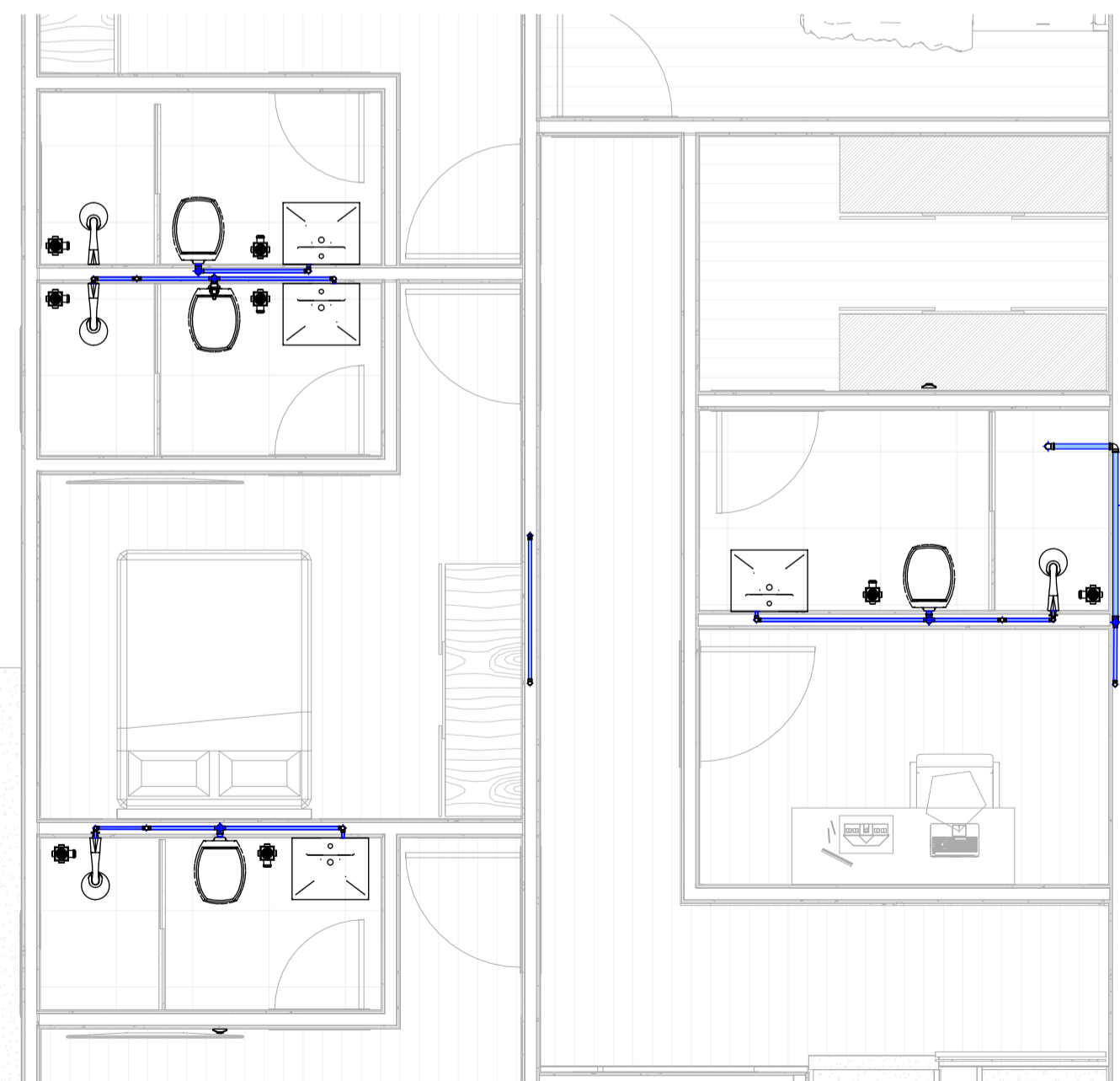
3 PAV. SUPERIOR 1 : 50
