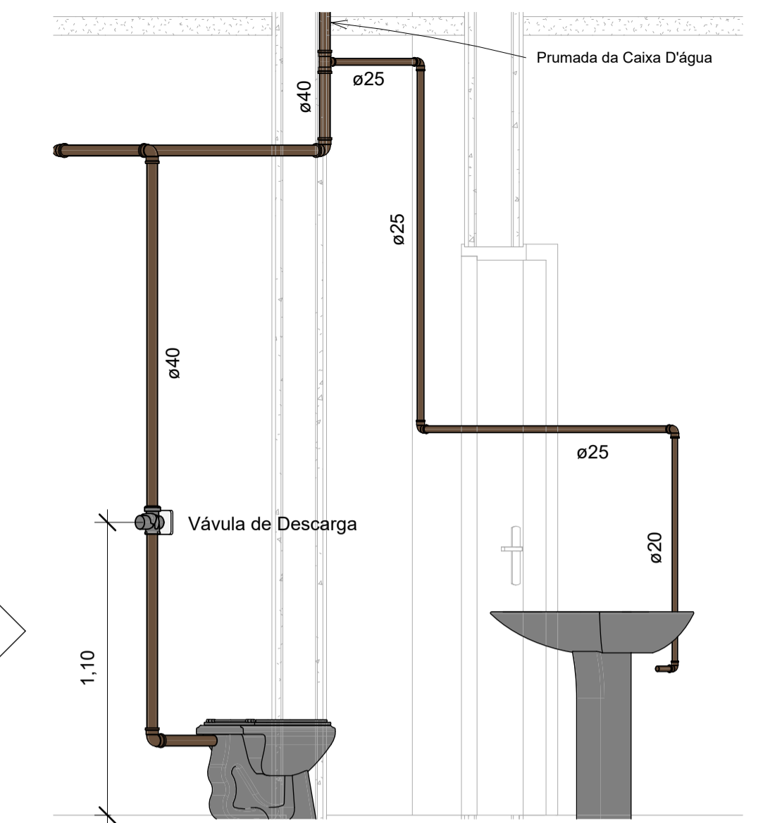
6 AF Lavabo Terreo 1 : 20
