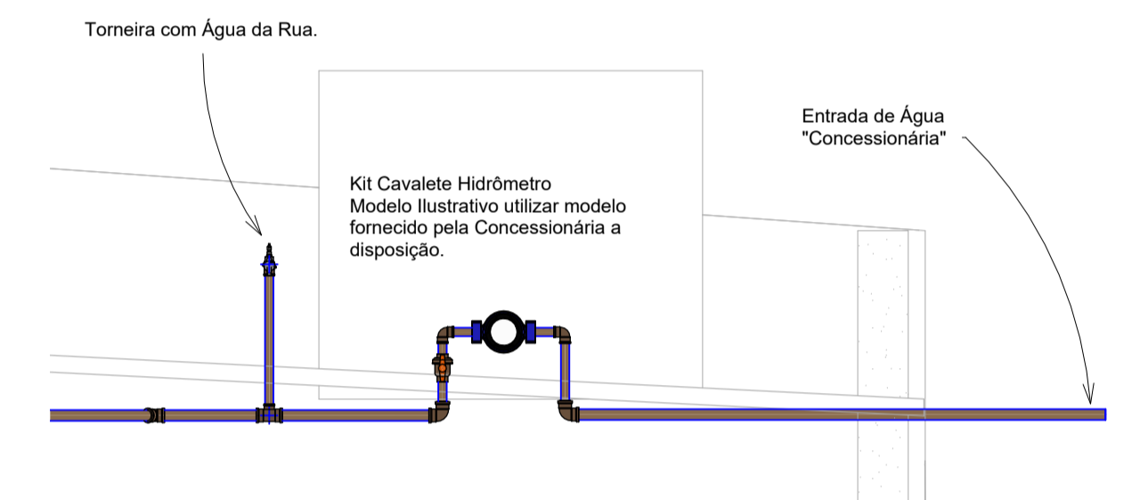
5 Entrada de Água 1 : 20
